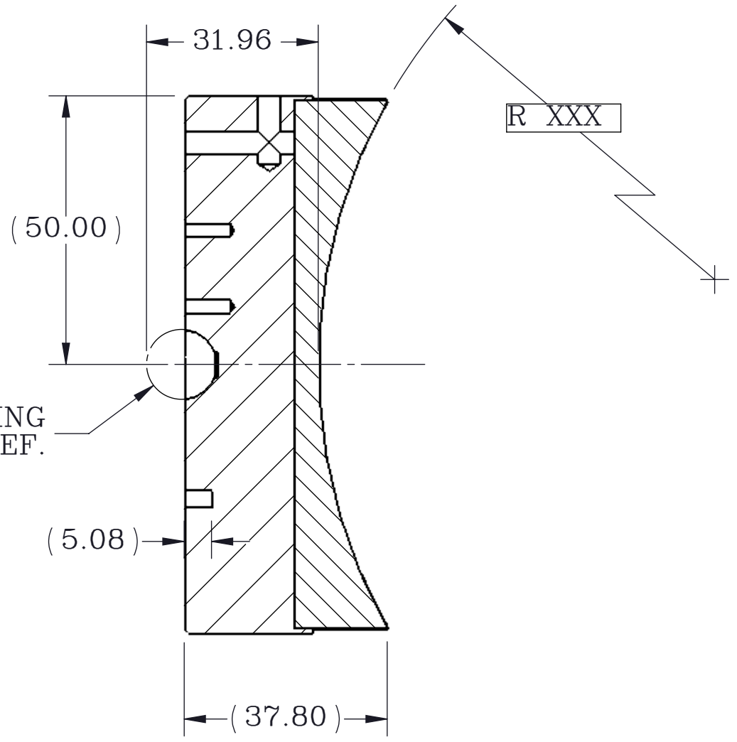
SECTION A-A
